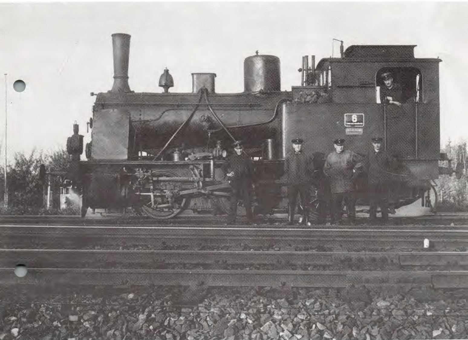
Naßdampf-Lokomotive v. Orenstein-Koppel anno 1913, welche damals zwischen Kaltenkirchen und Neumünster hin und her „dampfte“ (s. S. 5). (Aufnahme: AKN)
